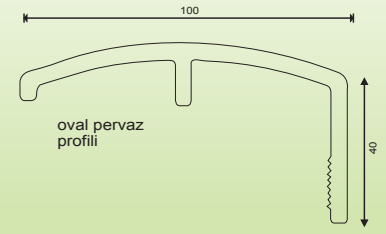
taç pervaz profili
